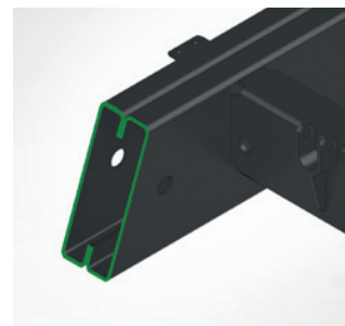
Dvojitý C rám podvozku
