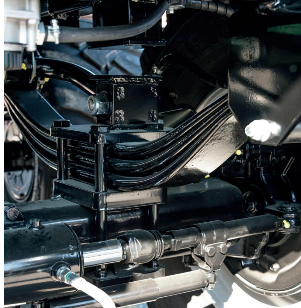
32 t pružinová jednotka se zesíle- nou vyrovnávací jednotkou
